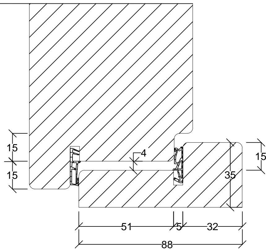
Drzwi 88 otwierane na zewnątrz
