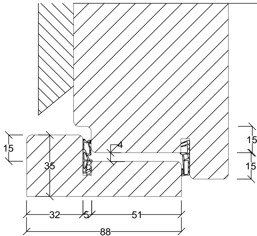
Drzwi 88 otwierane do wewnątrz
