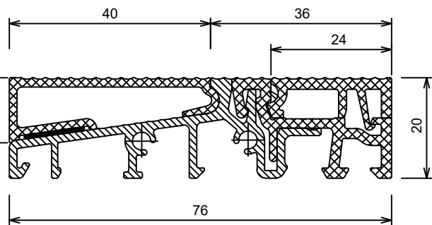
Türschwelle mit Trennprofil und PVC-Fülleiste TS57622-24-FL mit Aufsatzprofil TSA5761 für aussenaufgehende Türen mit Klebeband:
